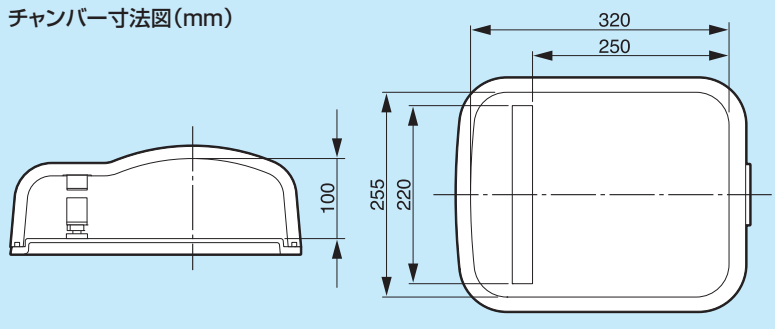
チャンバー寸法図(mm)
