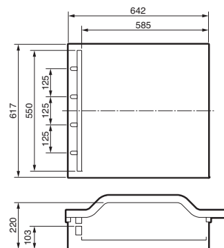
チャンバー寸法図(mm)
